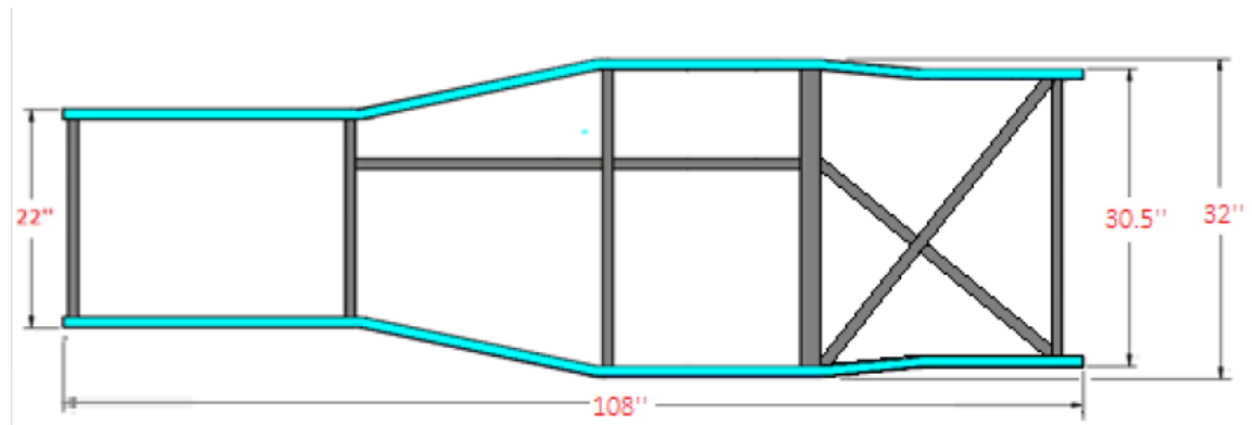
Figure 9 Mesure de la base châssis coupé
