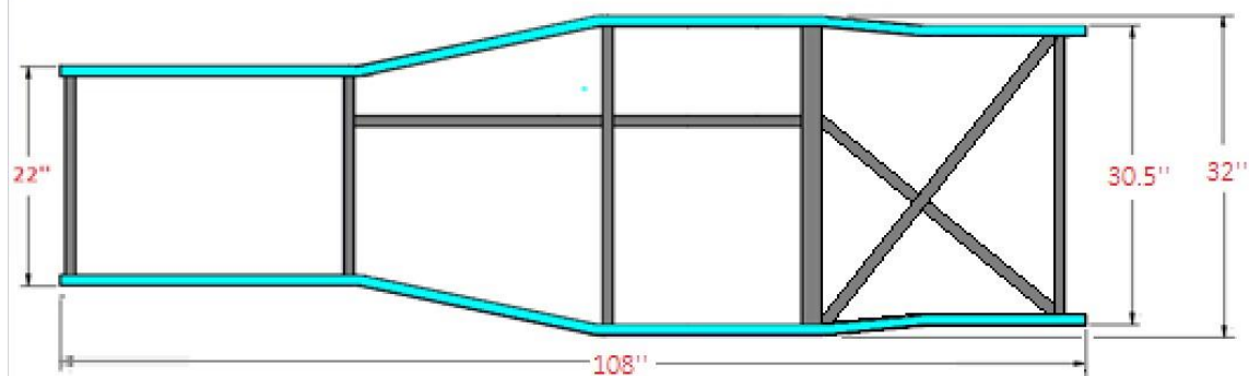
Figure 9 Mesure de la base châssis coupé
